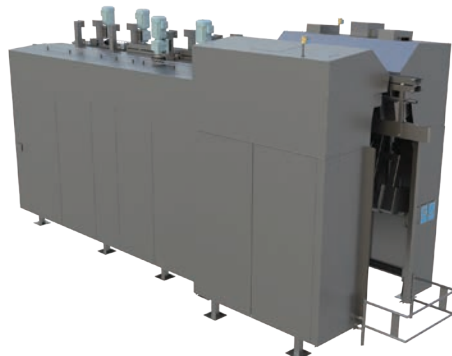
猪头和猪后蹄抛光机 (上图) 猪头和猪后蹄抛光以及6立轴和6横轴鞭打机
